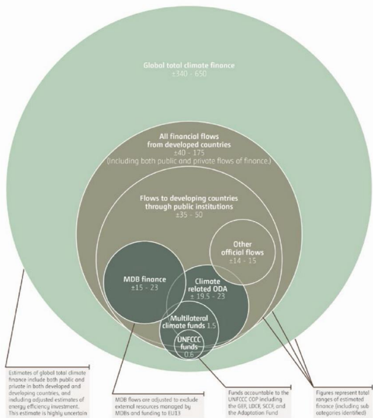
Graphique 8 Les financements climat en 2014 sont compris entre 340 et 650 Mds$
